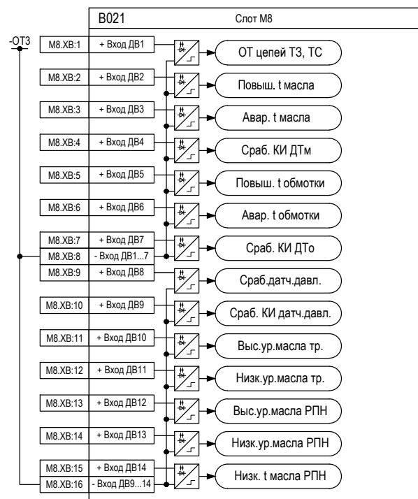
Рисунок Г.3 – Подключение дискретных входов и выходов к внутренним сигналам алгоритмов для блоков в слотах М6-М8
